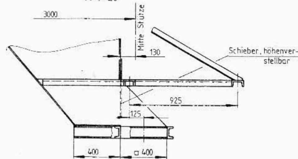
Motorplatte Kreiselbrecher M 1:20
