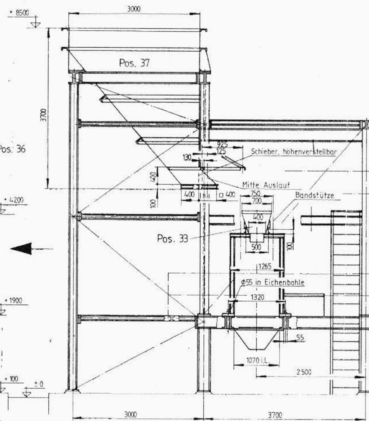
Siloauslauf M 1:20
