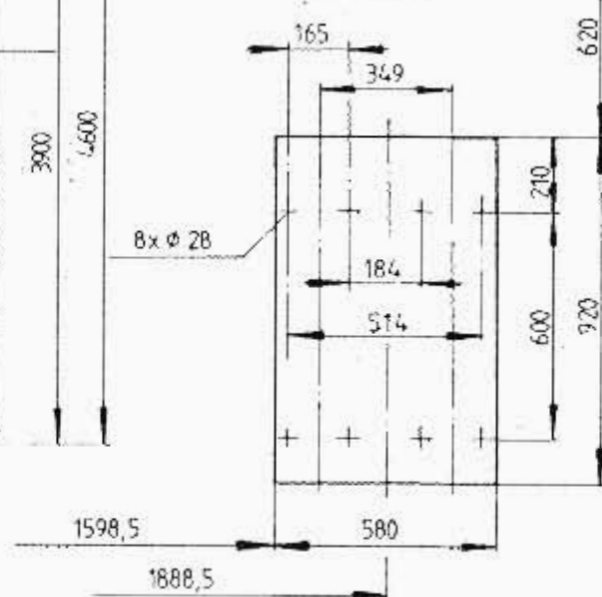
Motorplatte Kreiselbrecher M 1:20
