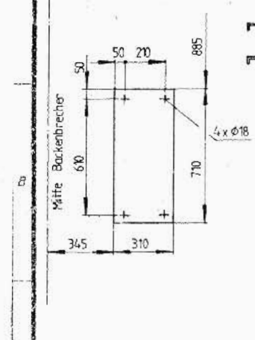
Motorplatte Backenbrecher M 1:20
