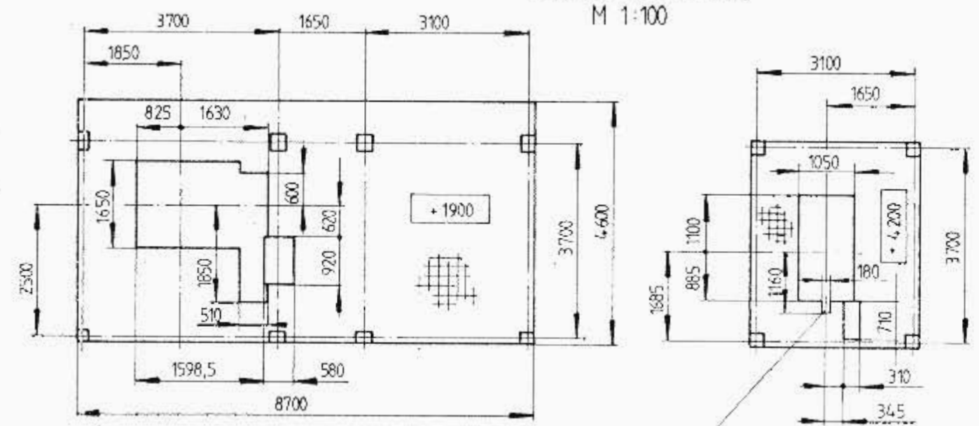
Gitterrostabdeckung M 1:100
